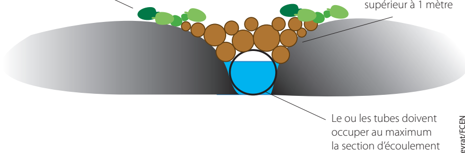
Dispositif de franchissement avec tuyaux PEHD
